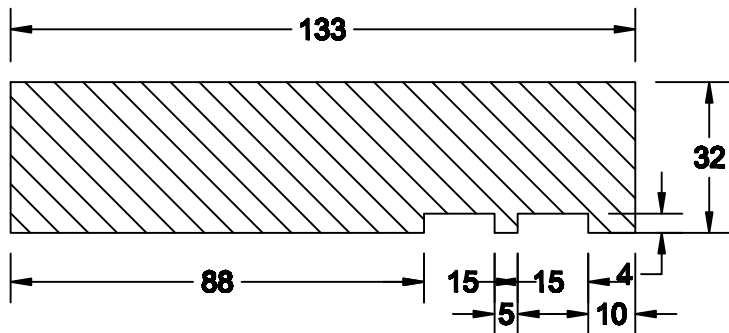
Profil Frame 32 x 133
