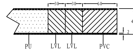
A-A
