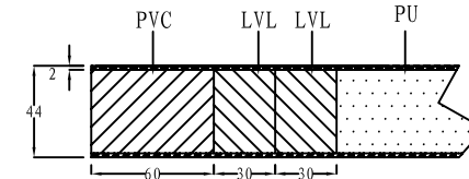
D-D
