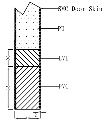
C-C
