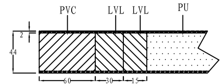
D-D
