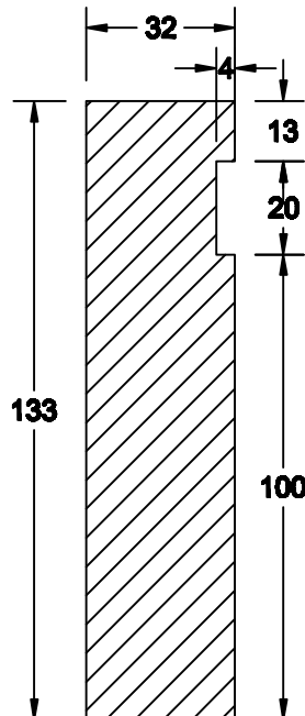
Profil Frame 32 x 133
