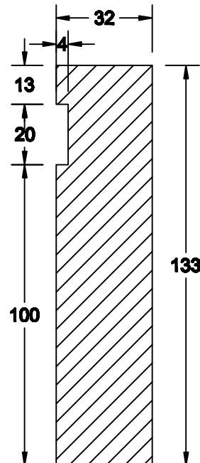
Profil Frame 32 x 133
