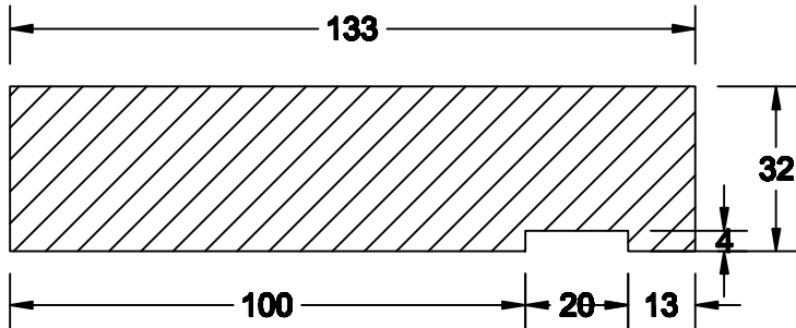
Profil Frame 32 x 133
