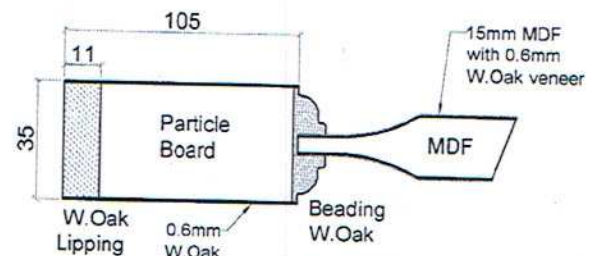
(SECTION-X) Construction Detail (Scale: N.T.S)
