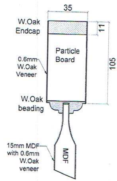
(SECTION-Y) Construction Detail (Scale: N.T.S)
