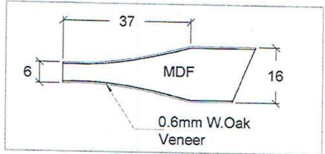
Sloupe Panel Detail (Scale: N.T.S)
