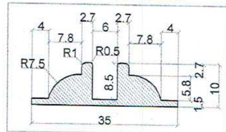
Sloupe Panel Detail (Scale: N.T.S)
